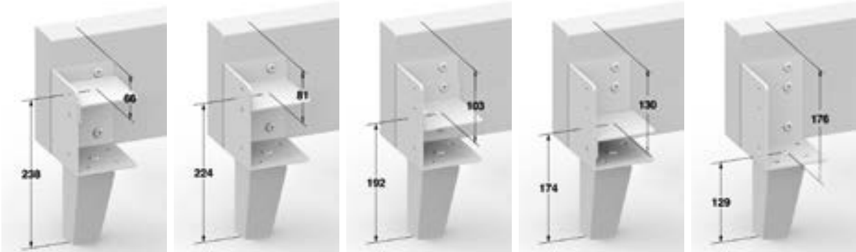
BEDFRAME H18, PIE4D H12 ARO DE CAMA H18, PIE4D. H12 - CADRE DE LIT H18, PIE4D. H12
