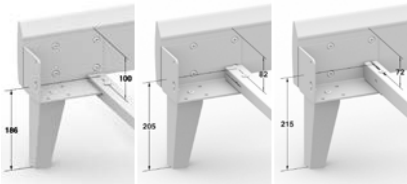
BEDFRAME H18, PIE4D H12 ARO DE CAMA H18, PIE4D. H12 - CADRE DE LIT H18, PIE4D. H12
