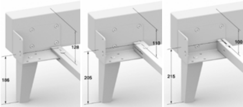
BEDFRAME H14 WITHOUT BED BASE, PIE6D. H17 ARO DE CAMA H14 SIN SOMIER, PIE6D. H17 - CADRE DE LIT H14 SANS SOMMIER, PIE6D. H17
