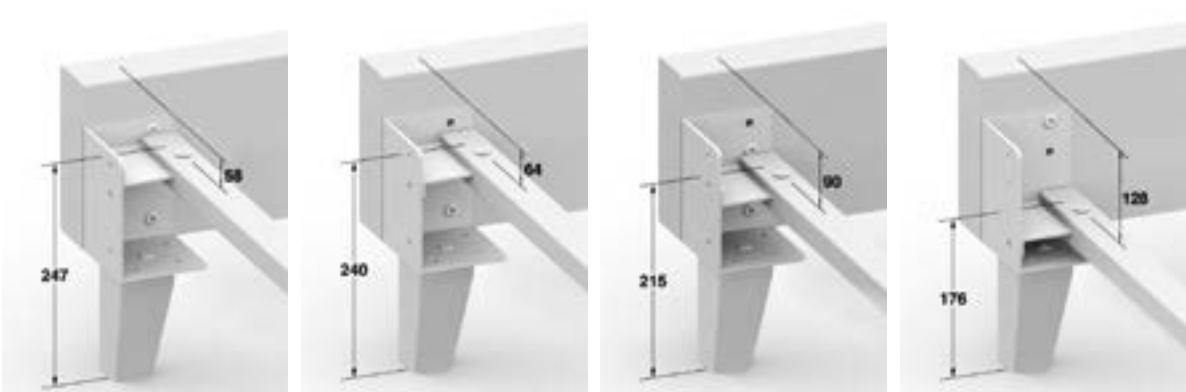
BEDFRAME H18 WITH HERCULES BRACKET, PIE4D H12 ARO DE CAMA H18 CON BARRA DE SUPORTE, PIE4D. H12 - CADRE DE LIT H18 AVEC BARRE DE SUPPORT, PIE4D. H12
